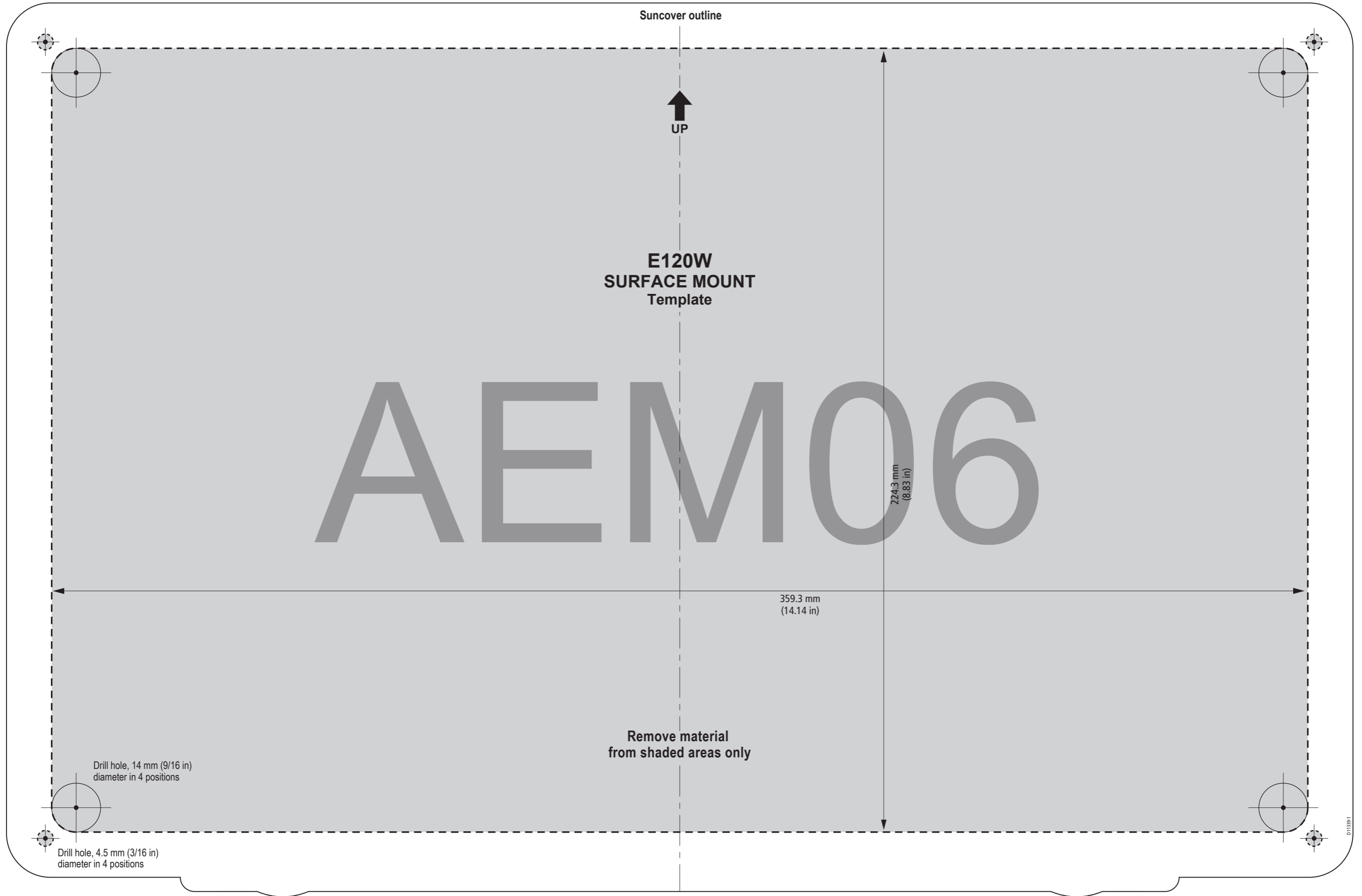
E120W Display surface mount template
